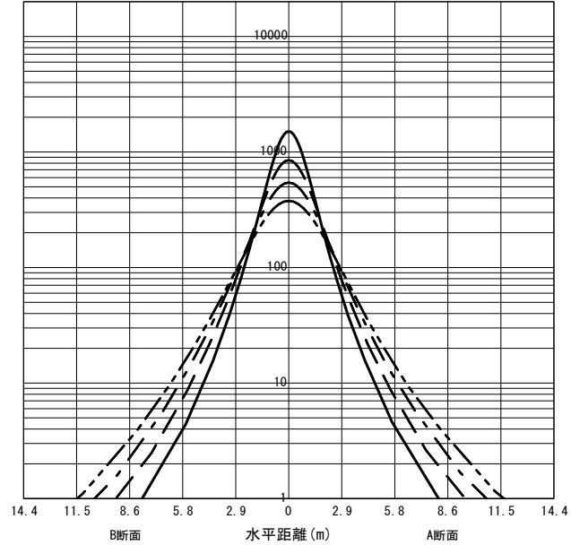
○直射水平面照度 (全光束: 9390 × 1 = 9390lm/台) 照度 (lx) — H1.50m --- H2.00m - - - H2.50m - · - · H3.00m (保守率: 1.00)
