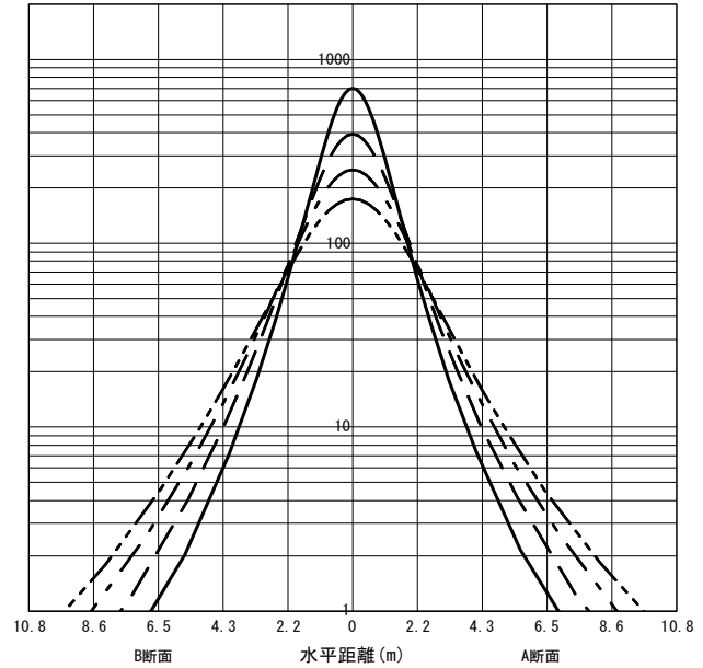
○直射水平面照度 (全光束: 4350 × 1 = 4350lm/台) 照度 (lx) — H1.50m --- H2.00m - - - H2.50m - · - · H3.00m (保守率: 1.00)
