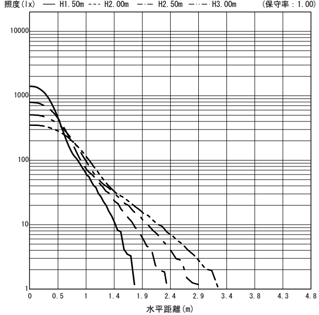
○直射水平面照度 (全光束: 1110 × 1 = 1110lm/台)
