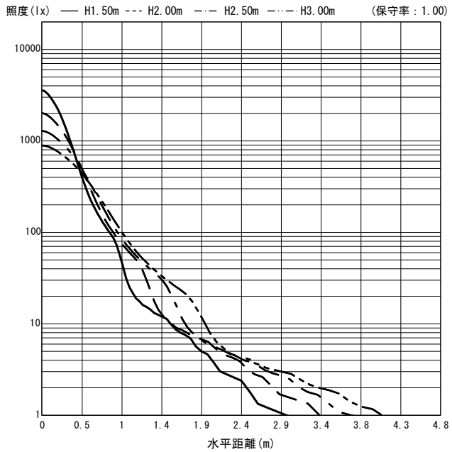
○直射水平面照度 (全光束: 1400 × 1 = 1400lm/台)
