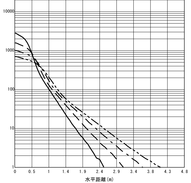
○直射水平面照度 (全光束：2070 × 1 = 2070lm/台) 照度 (lx) — H1.50m --- H2.00m - - - H2.50m - · - - H3.00m (保守率：1.00)
