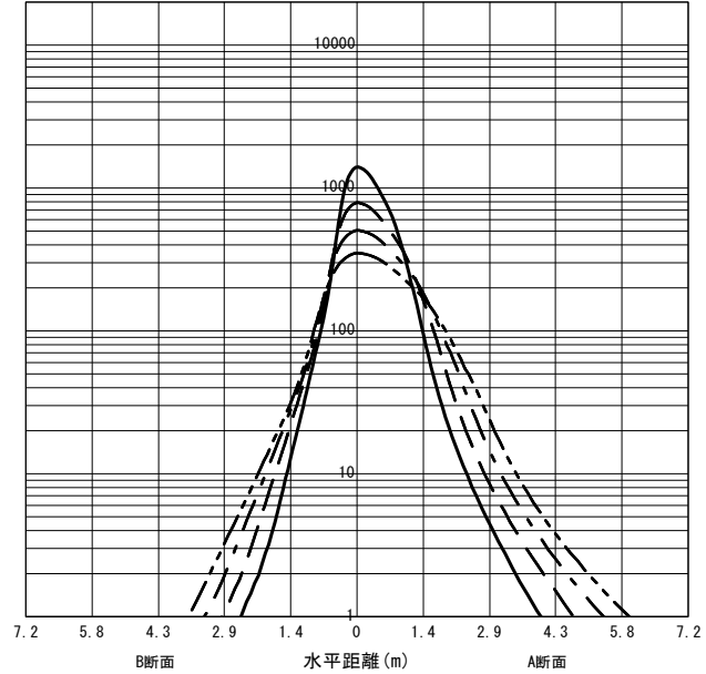
○直射水平面照度 (全光束: 1985 × 1 = 1985lm/台) 照度 (lx) — H1.50m --- H2.00m - - - H2.50m - · - - H3.00m (保守率: 1.00)
