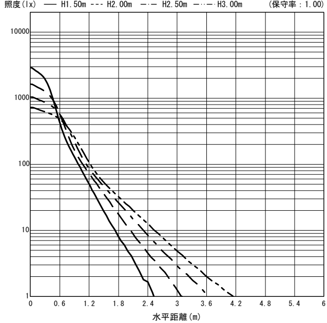
○直射水平面照度 (全光束: 2140 × 1 = 2140lm/台)
