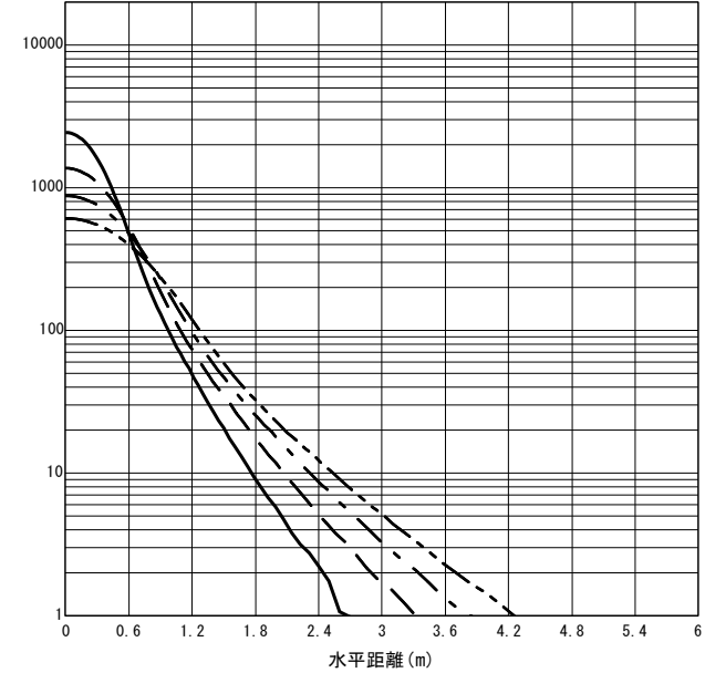
○直射水平面照度 (全光束: 2020 × 1 = 2020lm/台) 照度 (lx) — H1.50m --- H2.00m - - - H2.50m - · - · H3.00m (保守率: 1.00)
