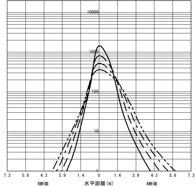
○直射水平面照度 (全光束: 2050 × 1 = 2050lm/台) 照度 (lx) — H1.50m --- H2.00m - - - H2.50m - · - · H3.00m (保守率: 1.00)
