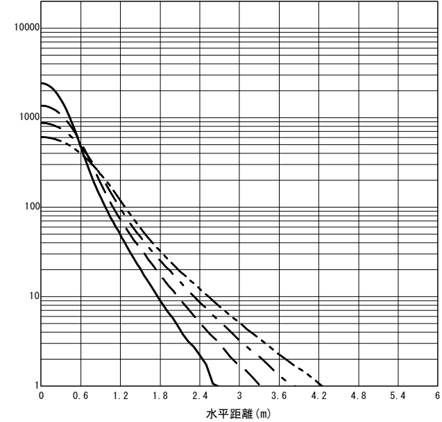
○直射水平面照度 (全光束: 2010 × 1 = 2010lm/台) 照度 (lx) — H1.50m --- H2.00m - - - H2.50m - · - · H3.00m (保守率: 1.00)
