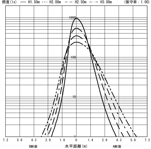
○直射水平面照度 (全光束: 2120 × 1 = 2120lm/台)
