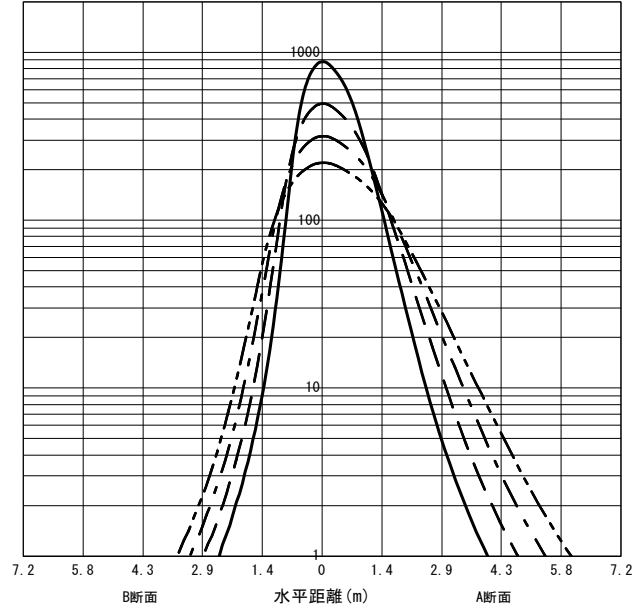
○直射水平面照度 (全光束: 1935 × 1 = 1935lm/台) 照度 (lx) — H1.50m --- H2.00m - - - H2.50m - · - · H3.00m (保守率: 1.00)
