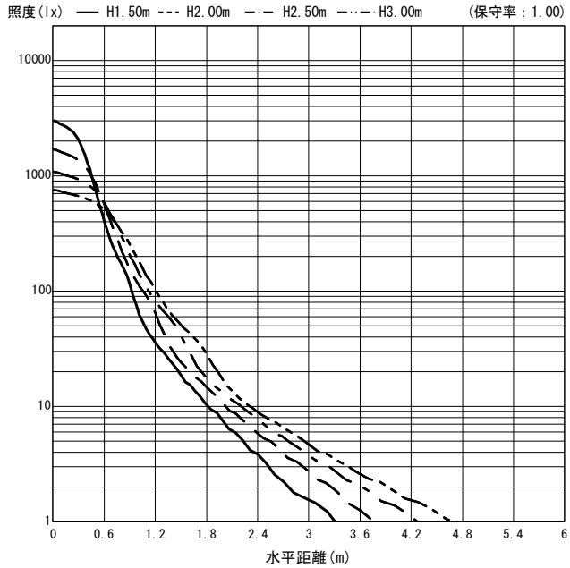
○直射水平面照度 (全光束: 2175 × 1 = 2175lm/台)
