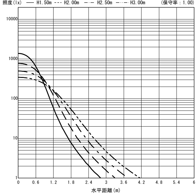
○直射水平面照度 (全光束 : 2085 × 1 = 2085lm/台)
