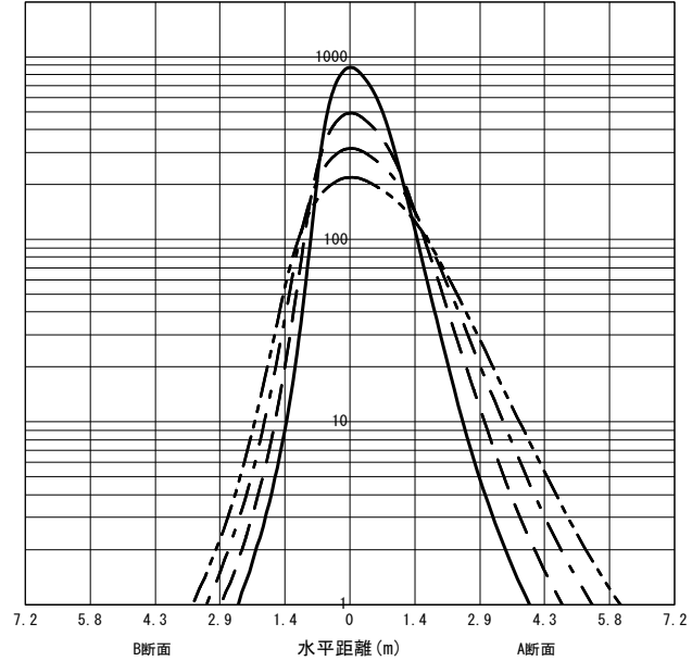
○直射水平面照度 (全光束: 1925 × 1 = 1925lm/台) 照度 (lx) — H1.50m --- H2.00m - - - H2.50m - · - · H3.00m (保守率: 1.00)
