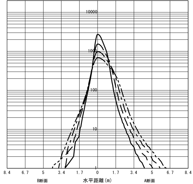
○直射水平面照度 (全光束: 2945 × 1 = 2945lm/台) 照度 (lx) — H1.50m --- H2.00m - - - H2.50m - · - · H3.00m (保守率: 1.00)
