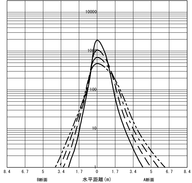
○直射水平面照度 (全光束: 2695 × 1 = 2695lm/台) 照度 (lx) — H1.50m --- H2.00m - - - H2.50m - · - · - H3.00m (保守率: 1.00)
