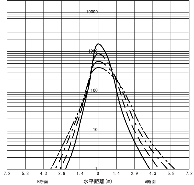
○直射水平面照度 (全光束 : 2225 × 1 = 2225lm/台) 照度 (lx) — H1.50m --- H2.00m - - - H2.50m - · - · H3.00m (保守率 : 1.00)
