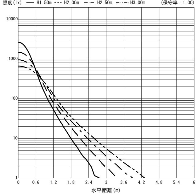
○直射水平面照度 (全光束: 2190 × 1 = 2190lm/台)
