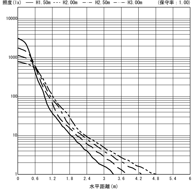
○直射水平面照度 (全光束: 2285 × 1 = 2285lm/台)
