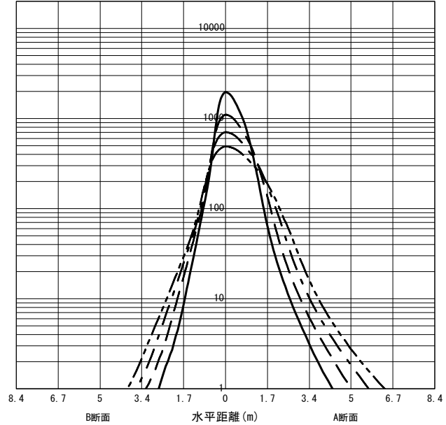
○直射水平面照度 (全光束: 2780 × 1 = 2780lm/台) 照度 (lx) — H1.50m --- H2.00m - - - H2.50m - · - · H3.00m (保守率: 1.00)
