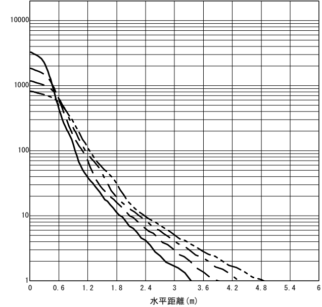
○直射水平面照度 (全光束: 2365 × 1 = 2365lm/台) 照度 (lx) — H1.50m --- H2.00m - - - H2.50m - · - · H3.00m (保守率: 1.00)
