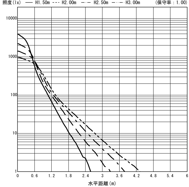
○直射水平面照度 (全光束: 2890 × 1 = 2890lm/台)
