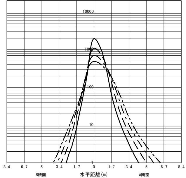
○直射水平面照度 (全光束 : 2770 × 1 = 2770lm/台) 照度 (lx) — H1.50m --- H2.00m - - - H2.50m - · - · H3.00m (保守率 : 1.00)
