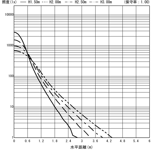
○直射水平面照度 (全光束 : 2255 × 1 = 2255lm/台)
