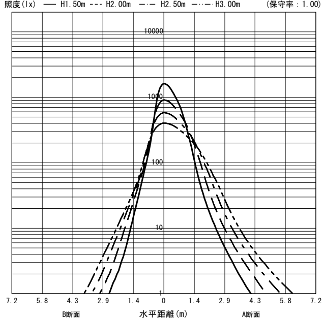
○直射水平面照度 (全光束: 2290 × 1 = 2290lm/台)
