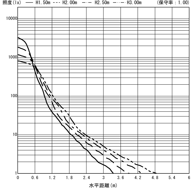
○直射水平面照度 (全光束: 2355 × 1 = 2355lm/台)
