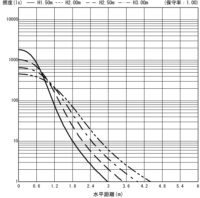
○直射水平面照度 (全光束: 2745 × 1 = 2745lm/台)
