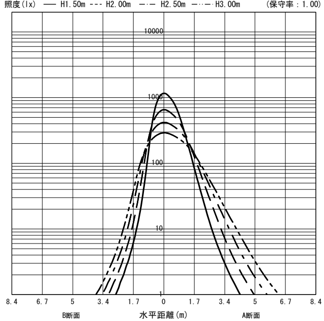
○直射水平面照度 (全光束 : 2550 × 1 = 2550lm/台)
