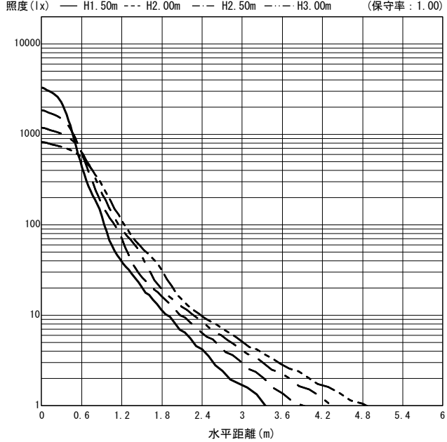
○直射水平面照度 (全光束: 2375 × 1 = 2375lm/台)
