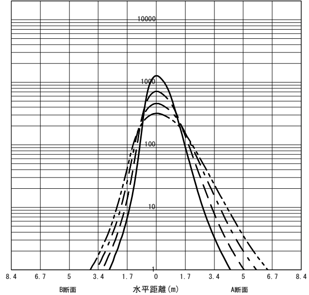
○直射水平面照度 (全光束: 2790 × 1 = 2790lm/台) 照度 (lx) — H1.50m --- H2.00m - - - H2.50m - · - · H3.00m (保守率: 1.00)
