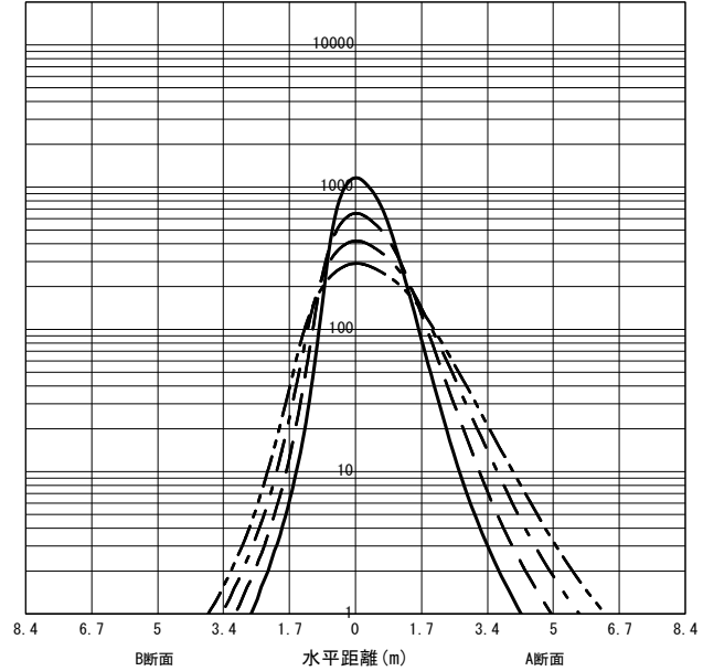
○直射水平面照度 (全光束: 2550 × 1 = 2550lm/台) 照度 (lx) — H1.50m --- H2.00m - - - H2.50m - · - · H3.00m (保守率: 1.00)
