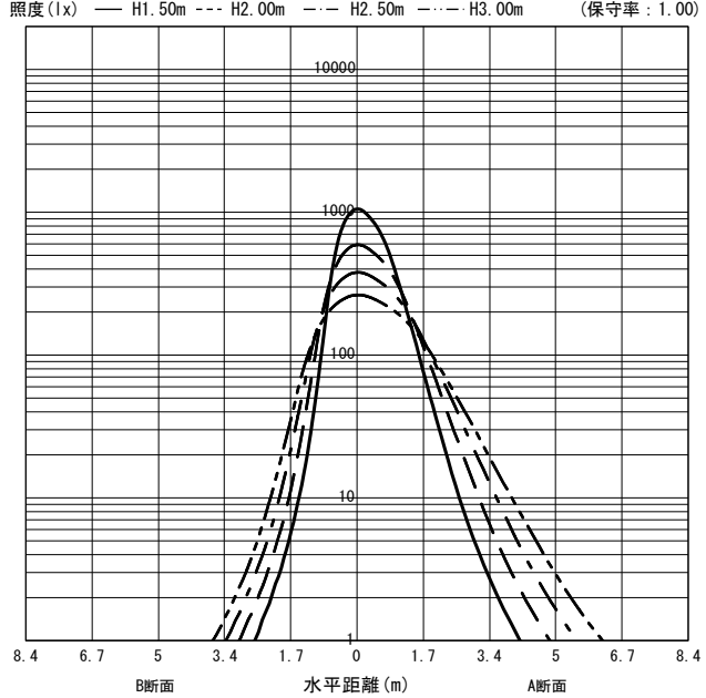
○直射水平面照度 (全光束 : 2310 × 1 = 2310lm/台)
