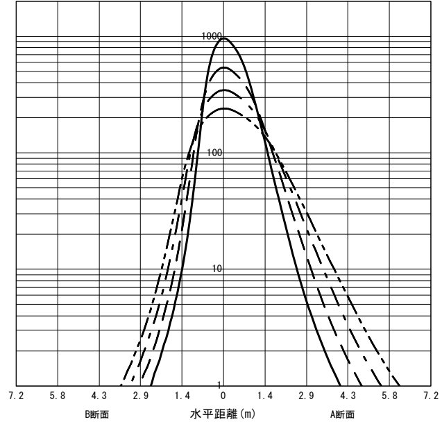
○直射水平面照度 (全光束: 2110 × 1 = 2110lm/台) 照度 (lx) — H1.50m --- H2.00m - - - H2.50m - · - · H3.00m (保守率: 1.00)
