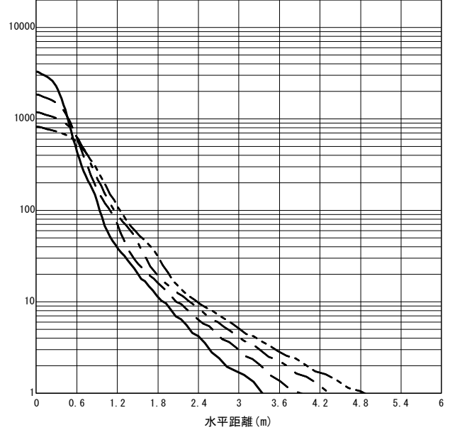
○直射水平面照度 (全光束: 2375 × 1 = 2375lm/台) 照度 (lx) — H1.50m --- H2.00m - - - H2.50m - · - · H3.00m (保守率: 1.00)
