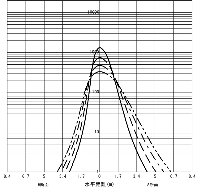
○直射水平面照度 (全光束: 2885 × 1 = 2885lm/台) 照度 (lx) — H1.50m --- H2.00m - - - H2.50m - · - · H3.00m (保守率: 1.00)
