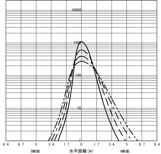
○直射水平面照度 (全光束: 2390 × 1 = 2390lm/台) 照度 (lx) — H1.50m --- H2.00m - - - H2.50m - · - · H3.00m (保守率: 1.00)
