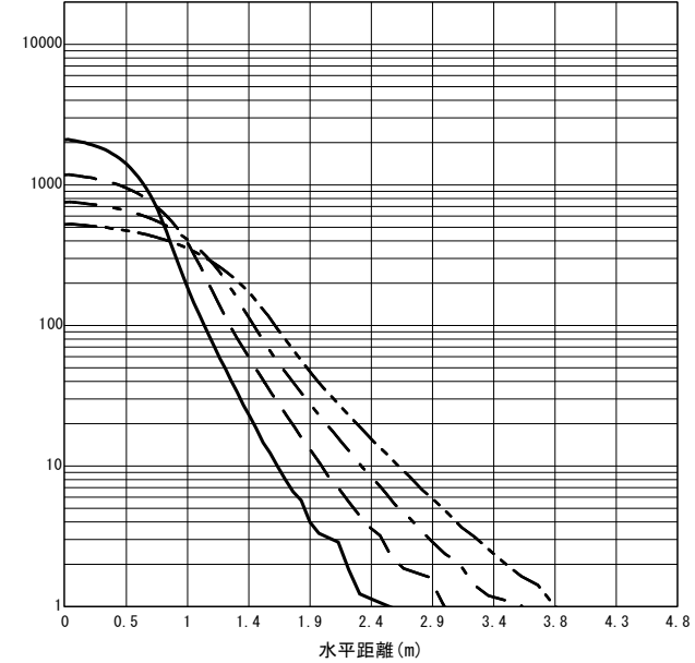
○直射水平面照度 (全光束: 3010 × 1 = 3010lm/台) 照度 (lx) — H1.50m --- H2.00m - - - H2.50m - · - · H3.00m (保守率: 1.00)
