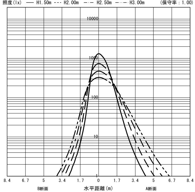
○直射水平面照度 (全光束 : 2880 × 1 = 2880lm/台)
