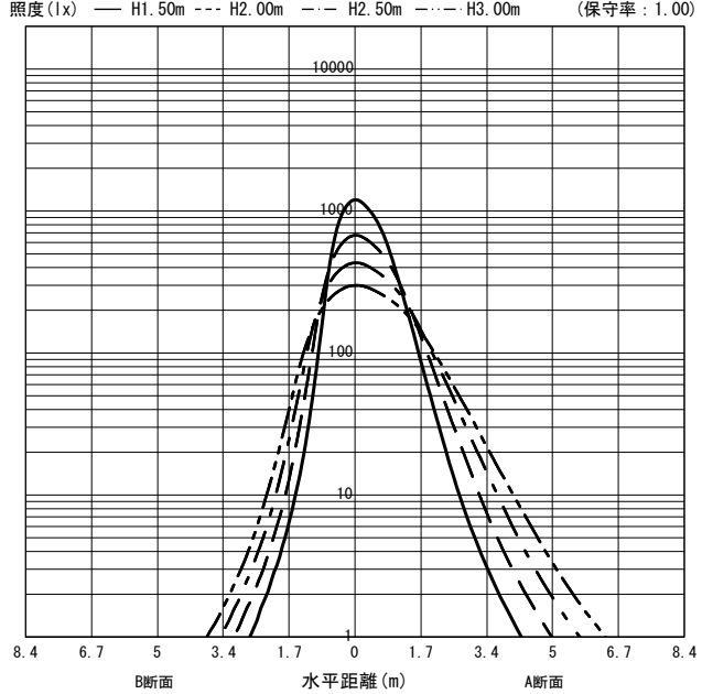
○直射水平面照度 (全光束 : 2630 × 1 = 2630lm/台)
