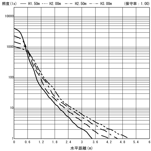
○直射水平面照度 (全光束 : 2955 × 1 = 2955lm/台)
