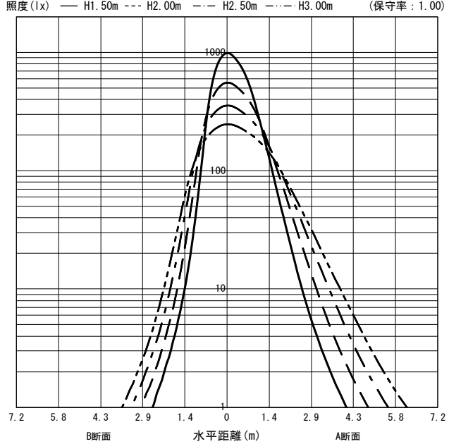
○直射水平面照度 (全光束: 2170 × 1 = 2170lm/台)
