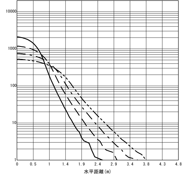
○直射水平面照度 (全光束: 3000 × 1 = 3000lm/台) 照度 (lx) — H1.50m --- H2.00m - - - H2.50m - · - · H3.00m (保守率: 1.00)
