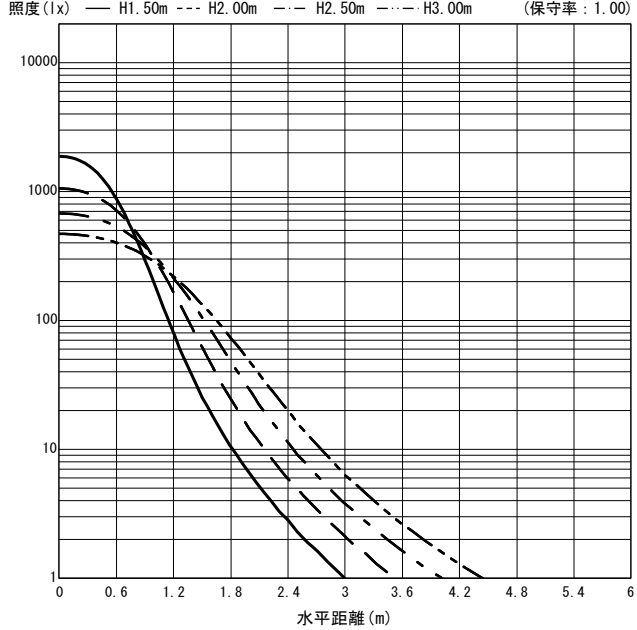
○直射水平面照度 (全光束: 2835 × 1 = 2835lm/台)
