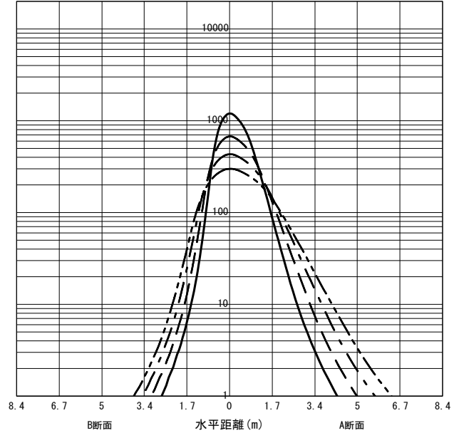
○直射水平面照度 (全光束: 2630 × 1 = 2630lm/台) 照度 (lx) — H1.50m --- H2.00m - - - H2.50m - · - · H3.00m (保守率: 1.00)
