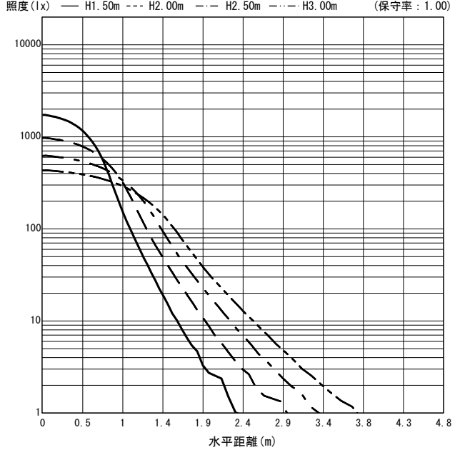
○直射水平面照度 (全光束: 2480 × 1 = 2480lm/台)
