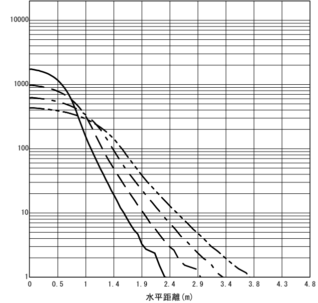
○直射水平面照度 (全光束: 2480 × 1 = 2480lm/台) 照度 (lx) — H1.50m --- H2.00m - - - H2.50m - · - · H3.00m (保守率: 1.00)
