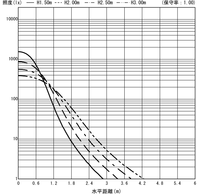
○直射水平面照度 (全光束: 2340 × 1 = 2340lm/台)
