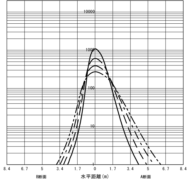
○直射水平面照度 (全光束 : 2380 × 1 = 2380lm/台) 照度 (lx) — H1.50m --- H2.00m - - - H2.50m - · - · H3.00m (保守率 : 1.00)
