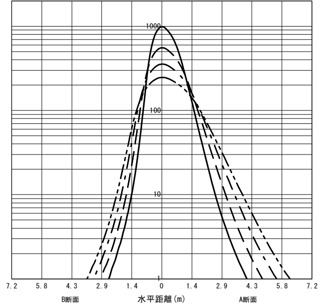
○直射水平面照度 (全光束: 2170 × 1 = 2170lm/台) 照度 (lx) — H1.50m --- H2.00m - - - H2.50m - · - · H3.00m (保守率: 1.00)
